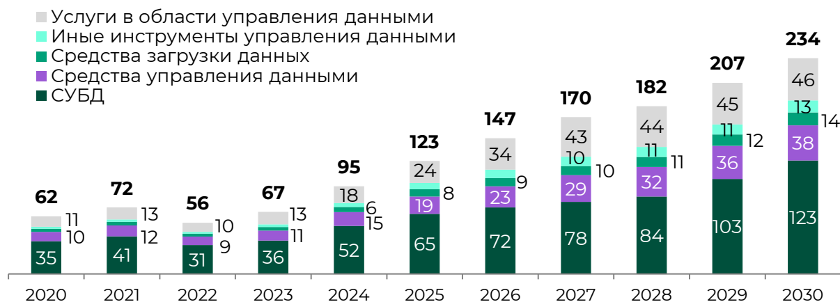
Рисунок 8. Прогноз динамики рынка СУБД и инструментов обработки данных по продуктам, млрд рублей. Источник: анализ ЦСР. Примечание: Данные за 2024–2030 гг. – прогноз.
